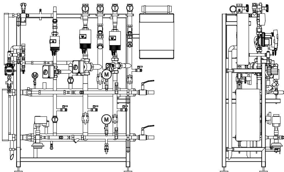
Typzusammensetzung am Beispiel der Wärmeübergabestation
